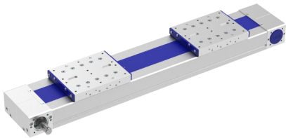
Kompakt-Lineareinheit HSB-delta®-ZSS-R-L
