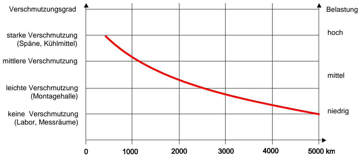
Bild 5: Nachschmierintervalle für die Kugelumlaufführung mit Kugelmutter
