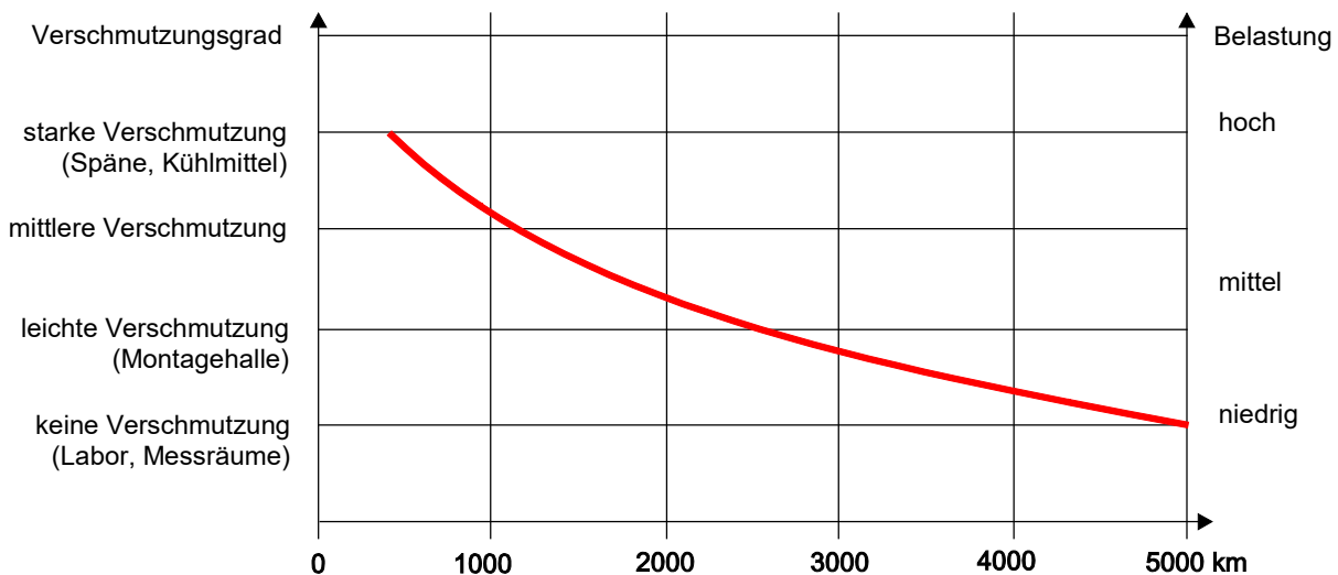
Bild 9: Nachschmierintervalle für die Kugelumlauführung mit Kugelkette
