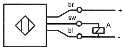
Schaltbild:
